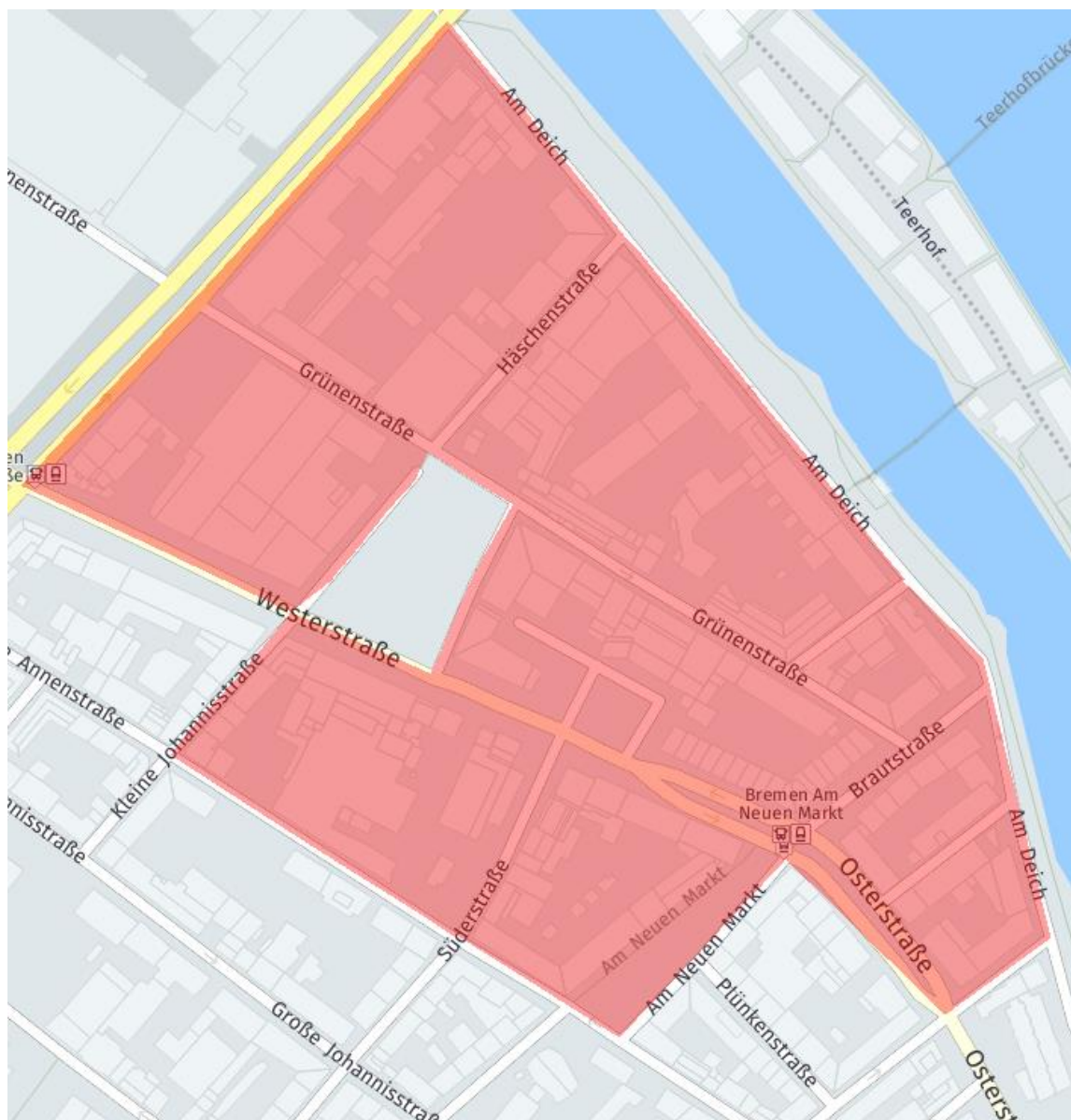
Karte der Stadt Bremen: Ausbaubereich entlang der Westerstraße
