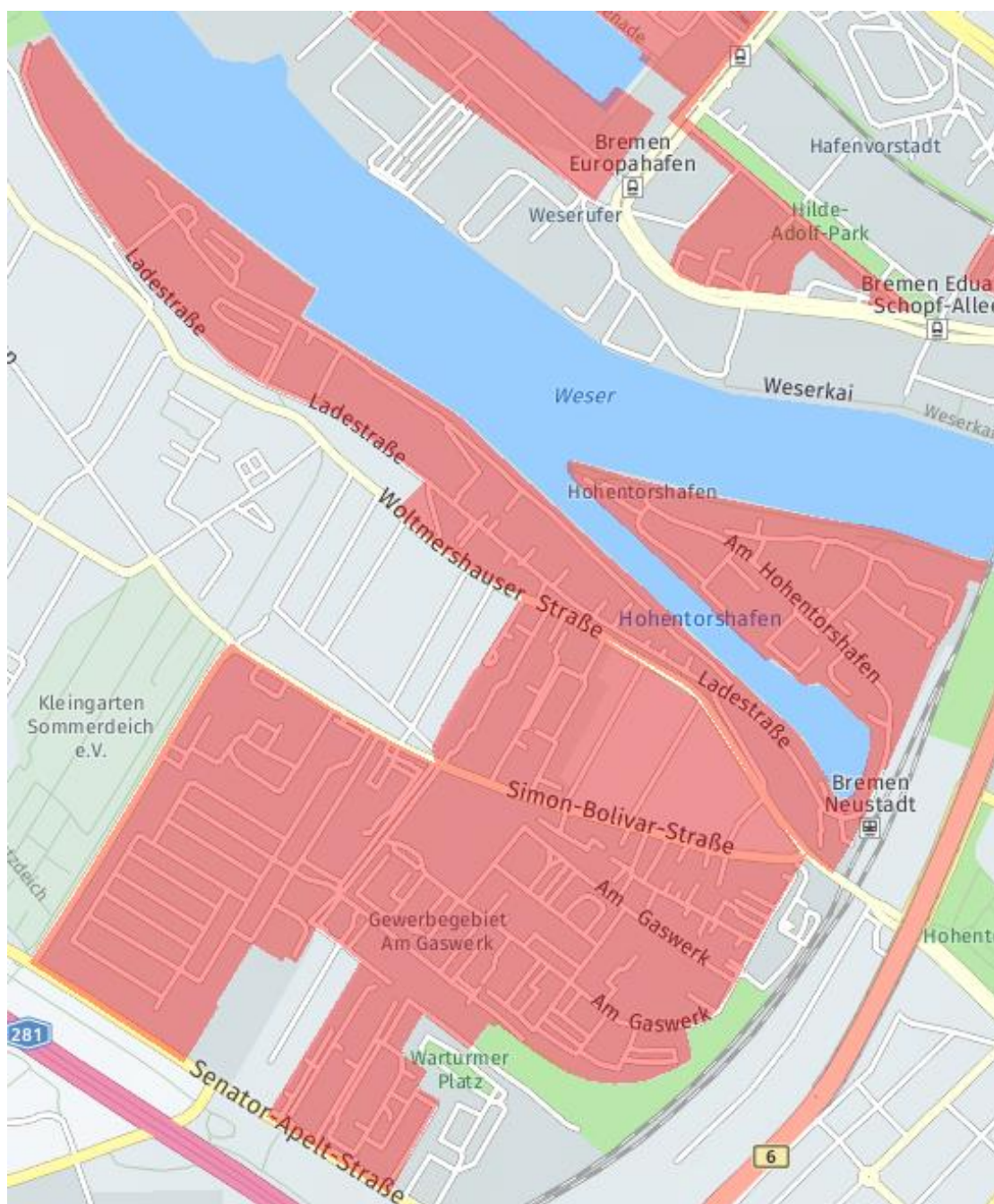
Karte der Stadt Bremen: Ausbaugelände im Gewerbegebiet Am Gaswerk und um den Hohentorshafen
