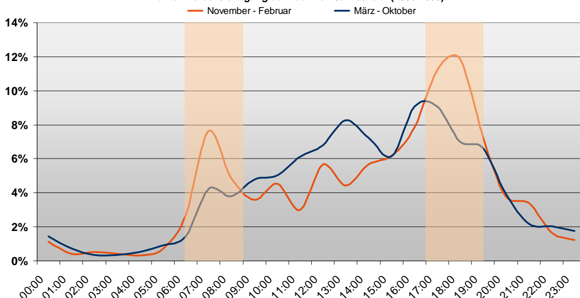
Tageszeitliche Verteilung der Fußgänger-Unfälle unter Berücksichtigung der "dunklen Jahreszeit" (2005-2009)
